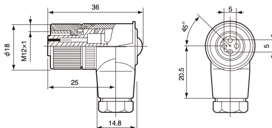
Conector Armable hembra M12 4 polos 90°
